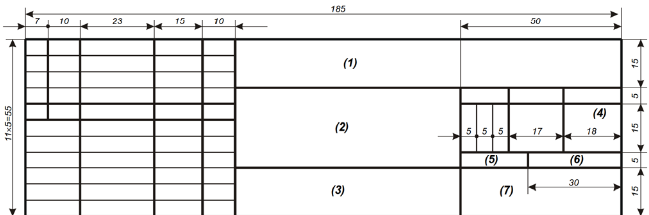
Рисунок 6.2 – Форма і розміри кутового штампу на кресленні
